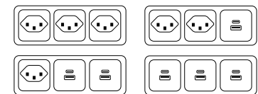
UnaK / UnaW mit Kabelführungskette oder Wing Steckdose T23, 230 V/16 A passend für Zargenhöhe M + K ab K500 3 x T23 / 2 x T23 + 1 x USB-A/C / 1 x T23 + 2 x USB-A/C / 3 x USB-A/C
